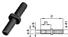
Adattatore a codolo portatubo
