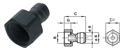
Adattatore femmina (a cono)
