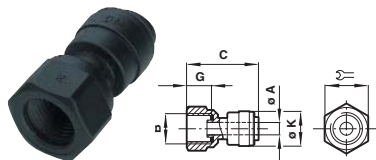
Adattatore femmina
