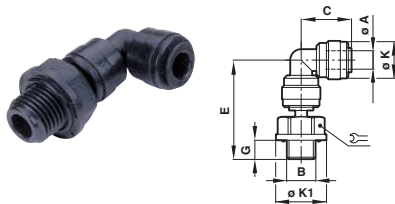
Gomito girevole 90°
