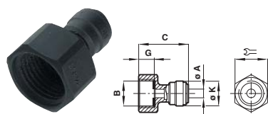
Adattatore femmina (di tipo piatto)
