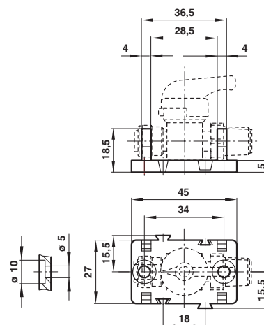
Clip di montaggio della valvola di esclusione (solo per valvole Ø 10)
